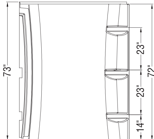
Mur C
